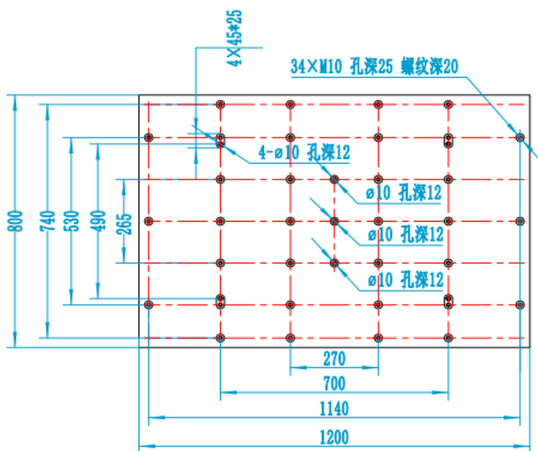
上台面连接尺寸
