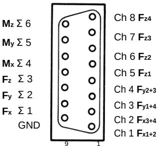
电荷放大器 8 个输出信号 加法器 6 个输出信号
