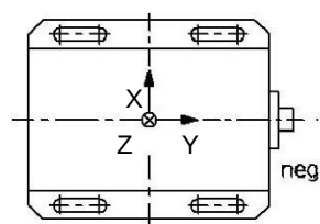
测力台 HR-FP3410
