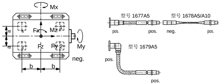
图 4: HR-FP3410 测量系统图例
