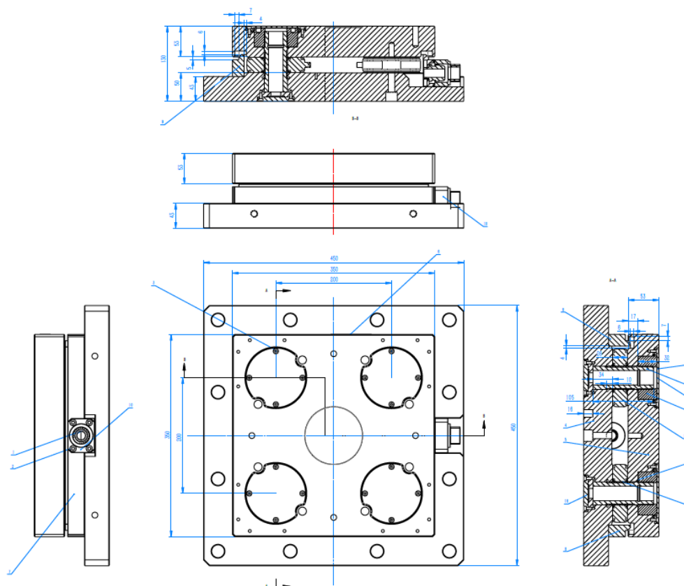
测力台 HR-FP3410
